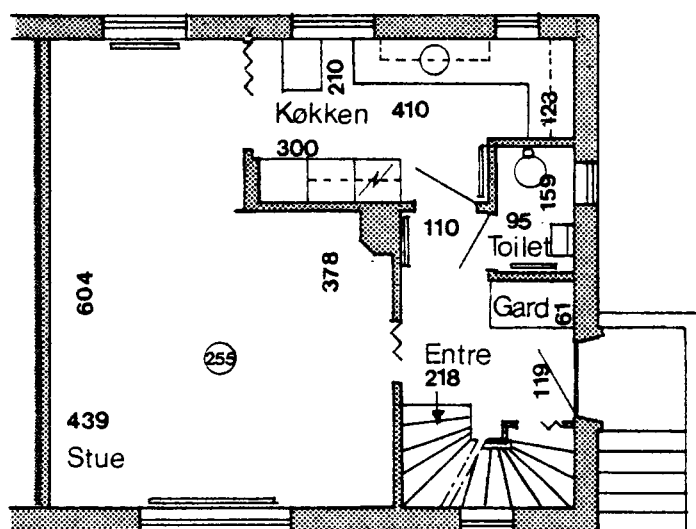
Stueplan
