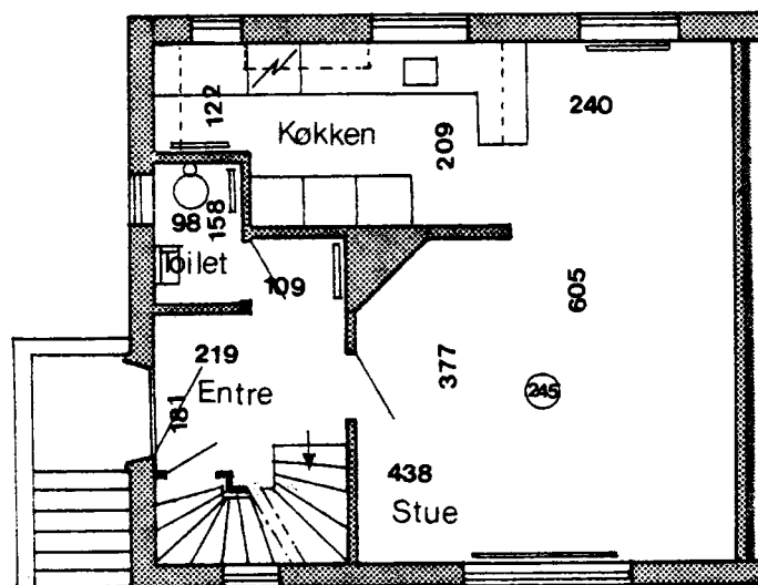
Stueplan
