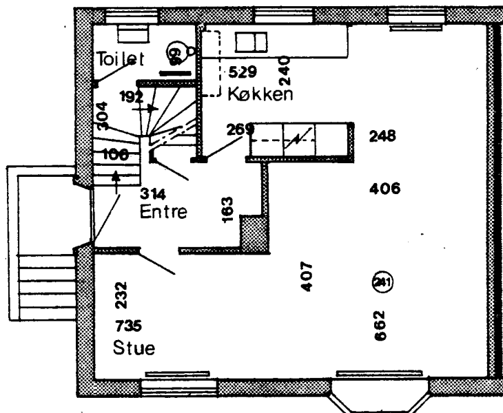
Stueplan
