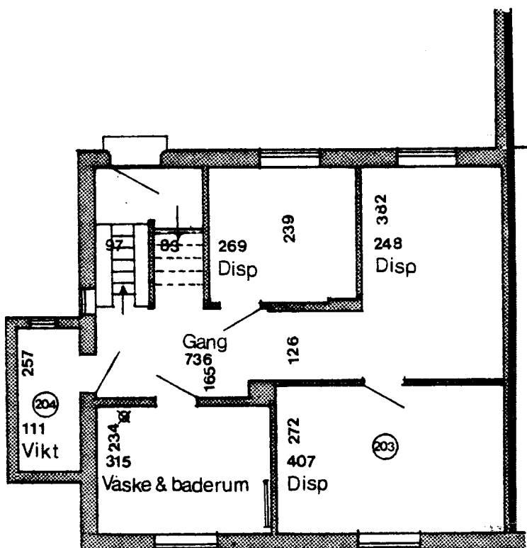
Kælderplan
