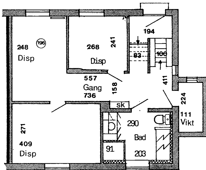
Kælderplan
