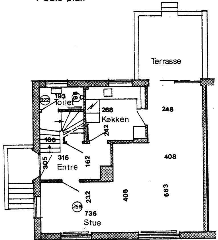
Stueplan
