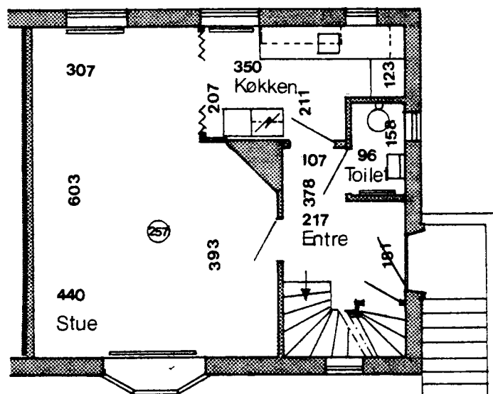
Stueplan
