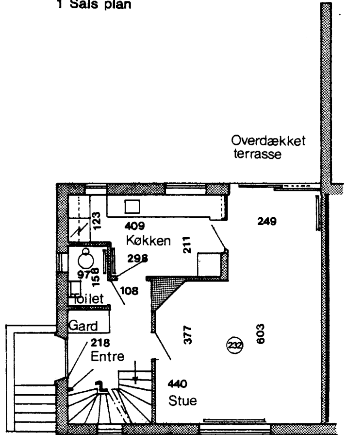
Stueplan
