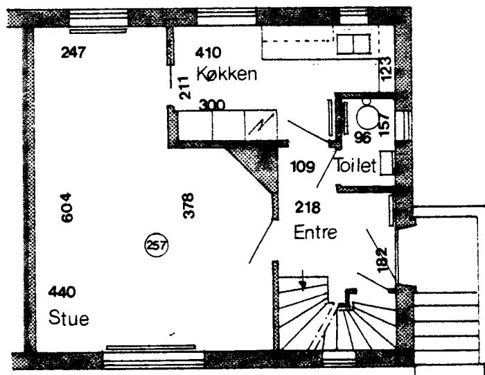
Stueplan
