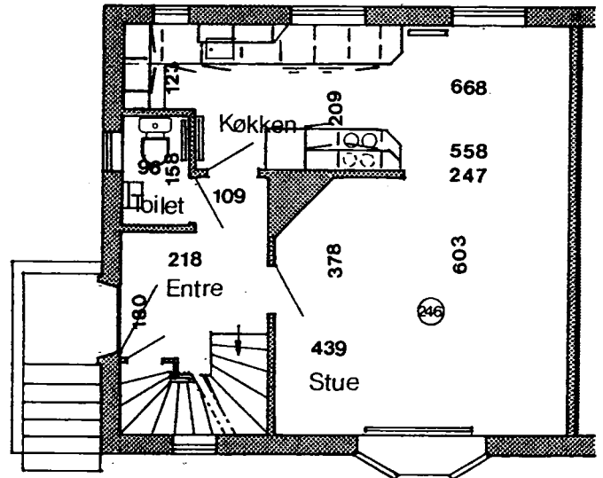
Stueplan
