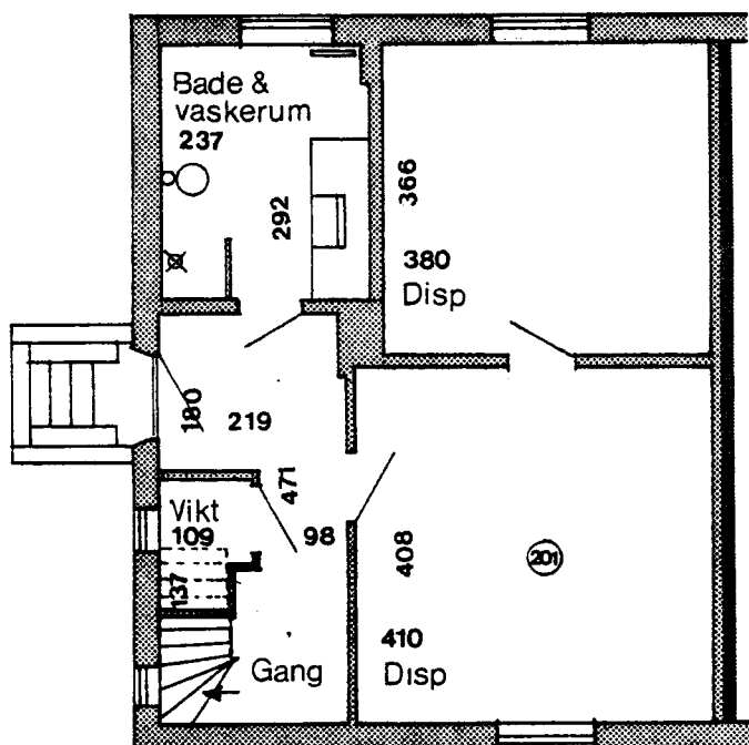
Kælderplan
