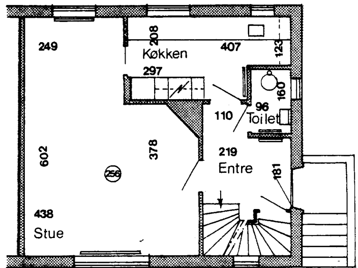
Stueplan
