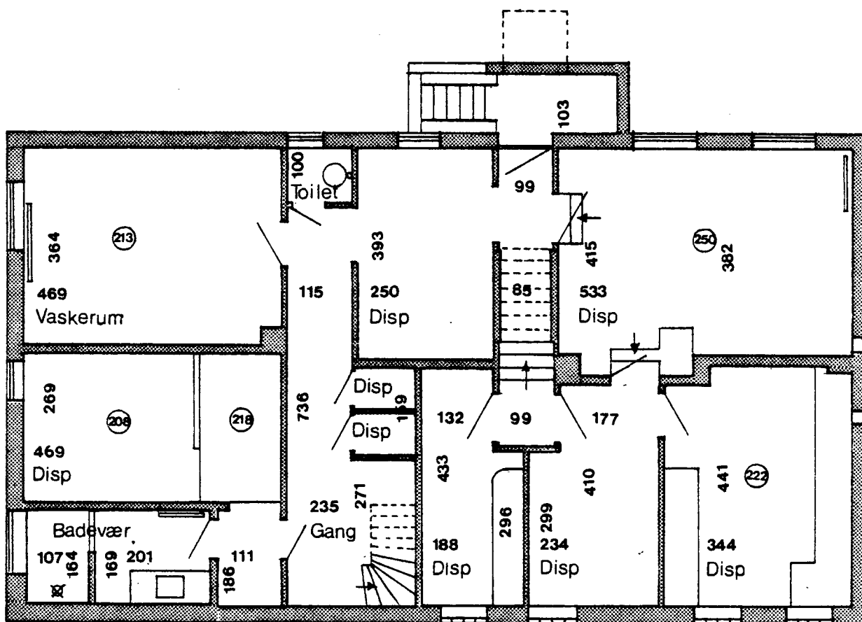
Kælderplan
