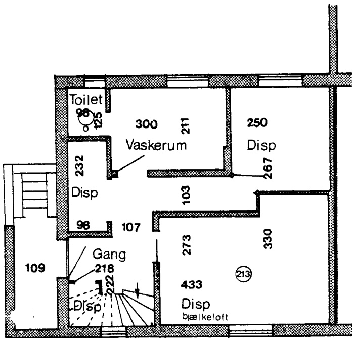
Kælderplan
