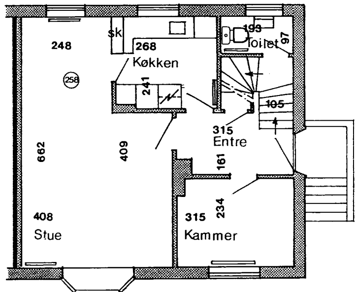
Stueplan
