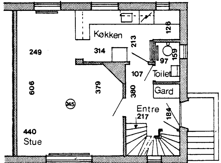
Stueplan
