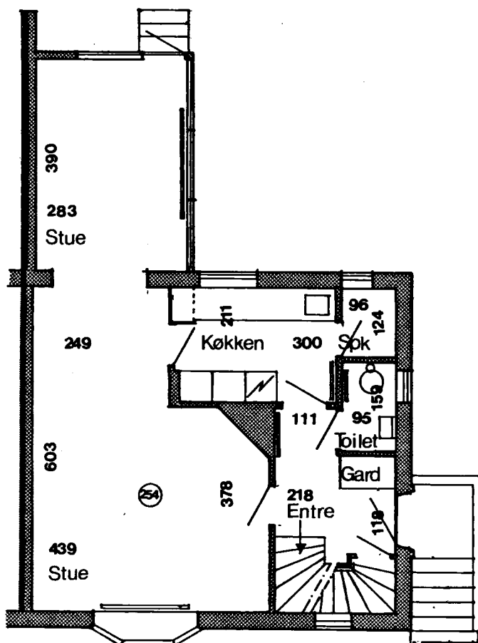
Stueplan
