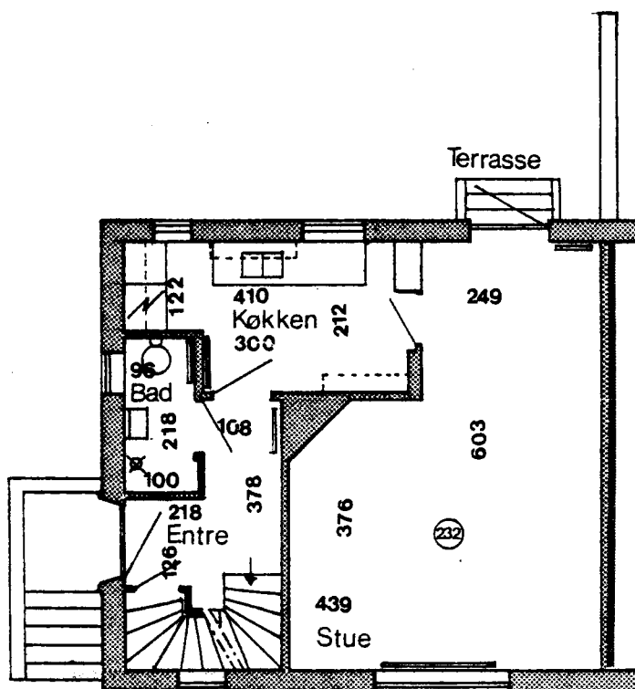
Stueplan
