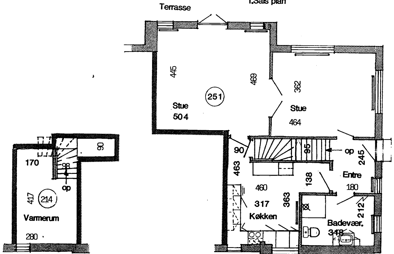
Kælderplan
