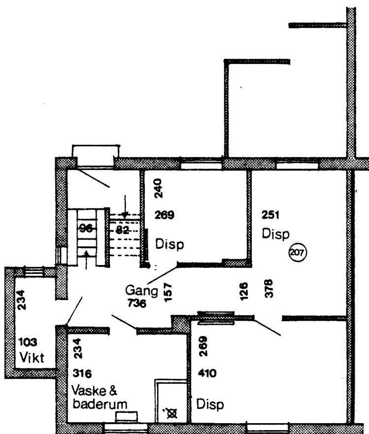
Kælderplan
