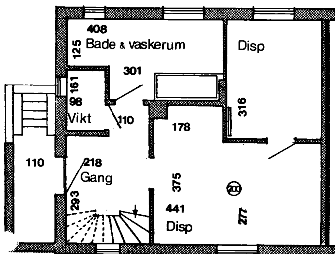
Kælderplan
