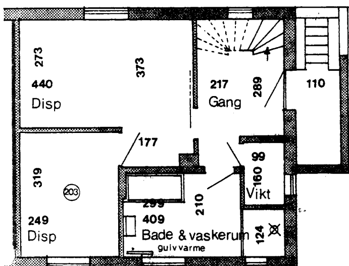
Kælderplan
