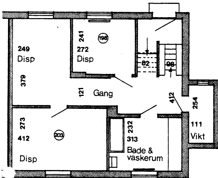
Kælderplan
