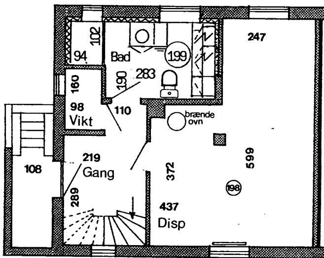
Kælderplan
