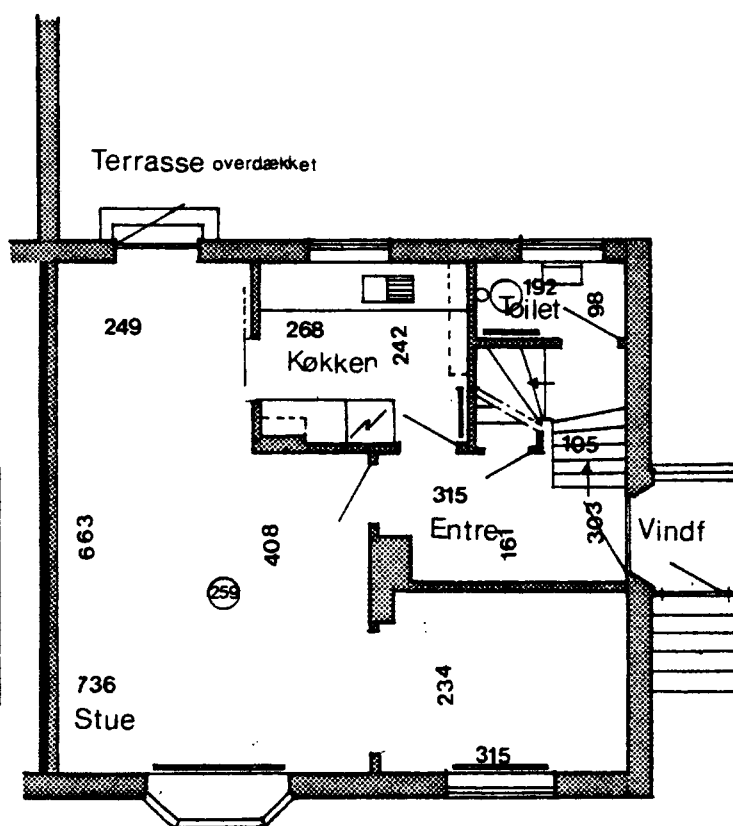
Stueplan
