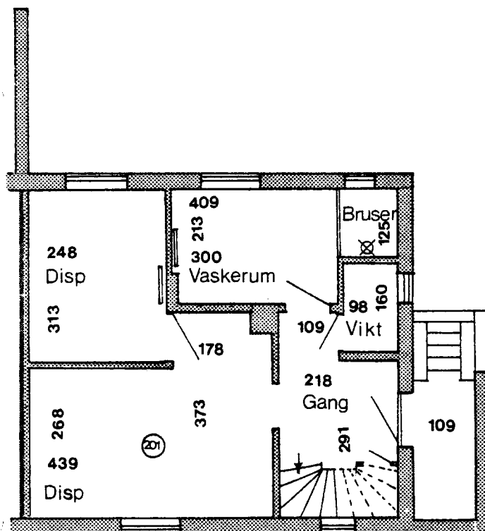
Kælderplan
