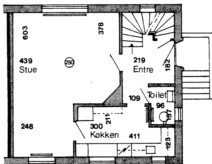
Stueplan
