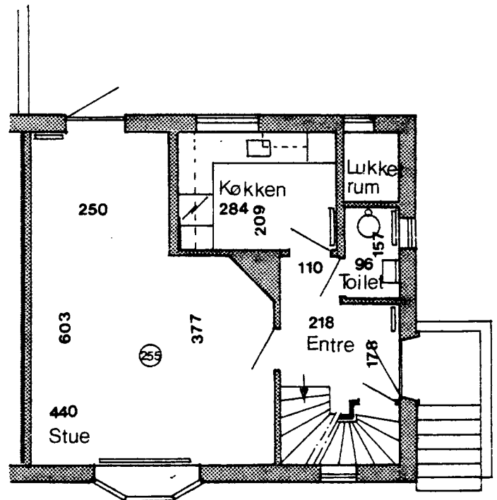
Stueplan
