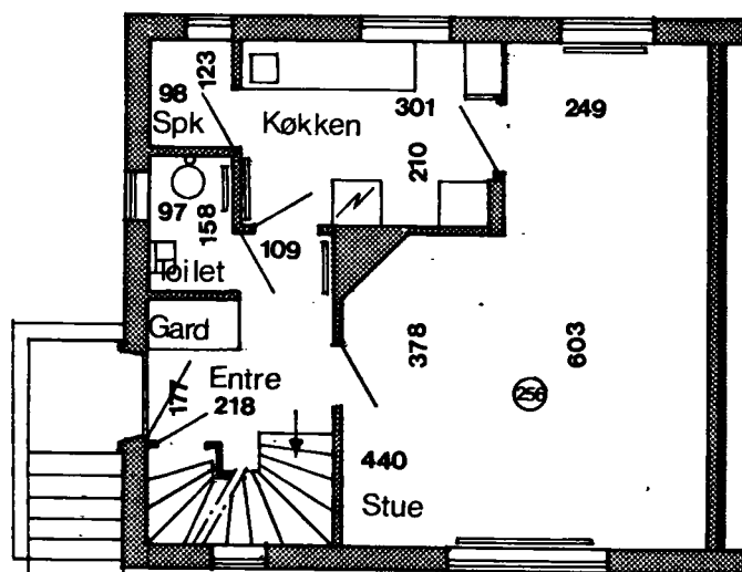
Stueplan
