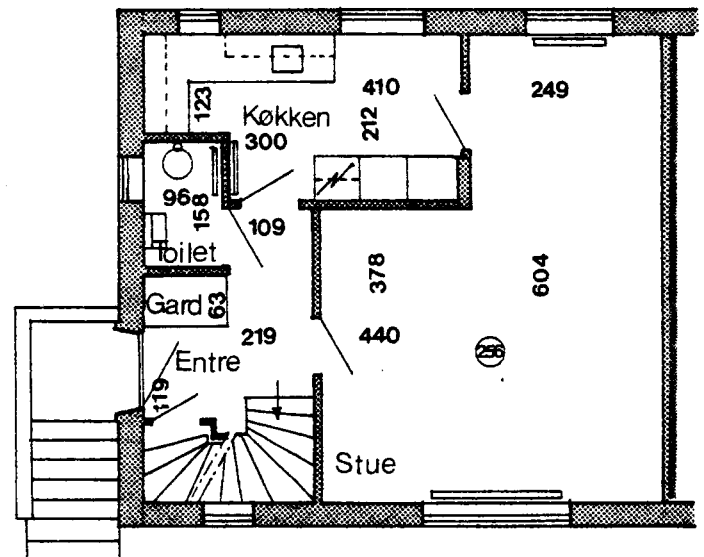
Stueplan
