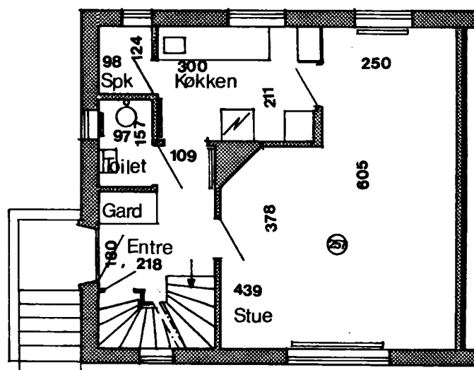
Stueplan
