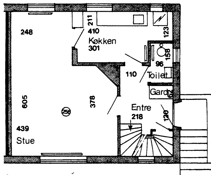
Stueplan
