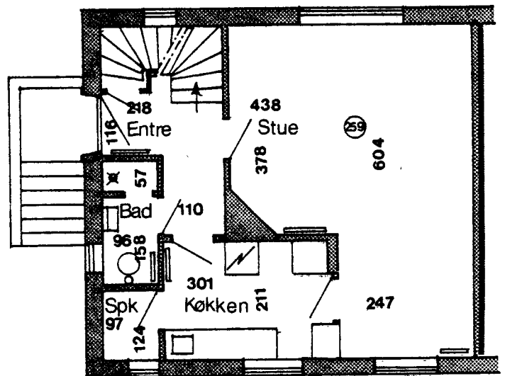
Stueplan
