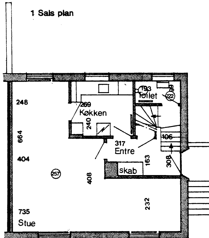
Stueplan
