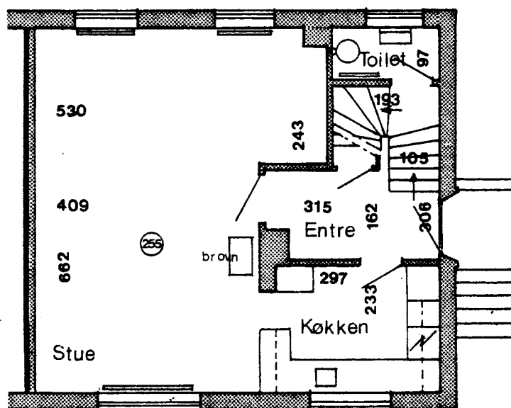
Stueplan
