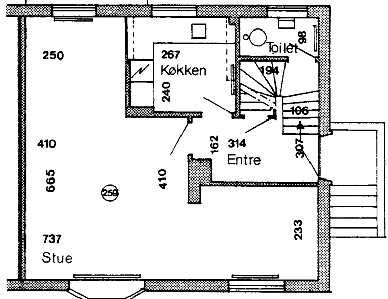
Stueplan
