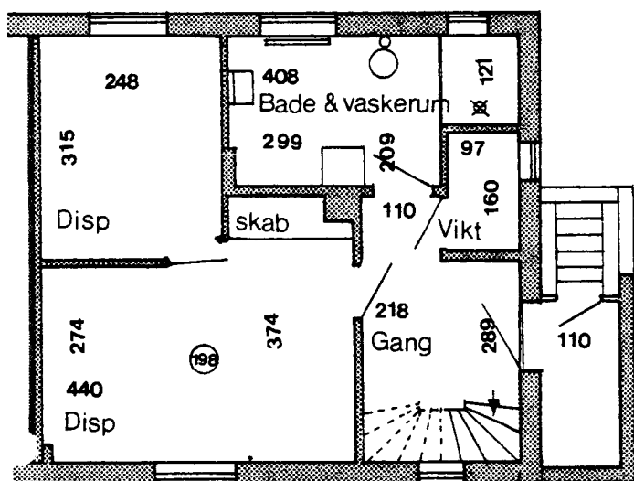
Kælderplan
