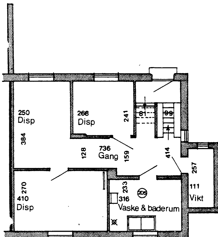
Kælderplan
