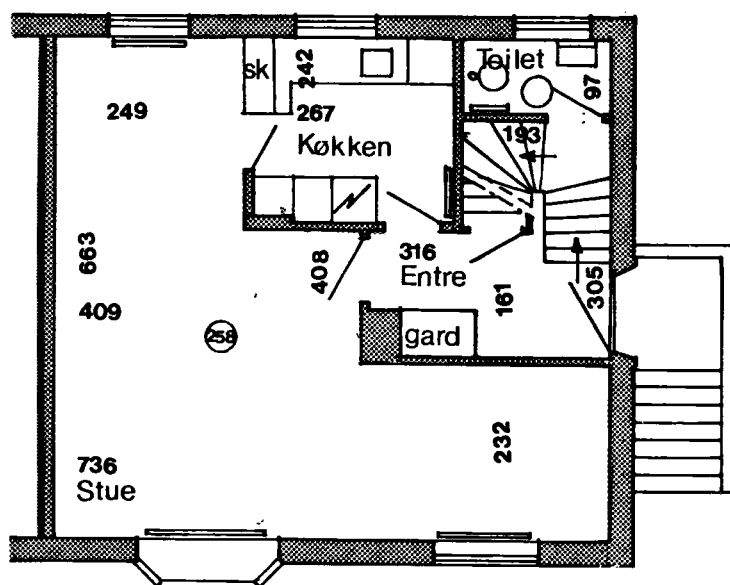
Stueplan
