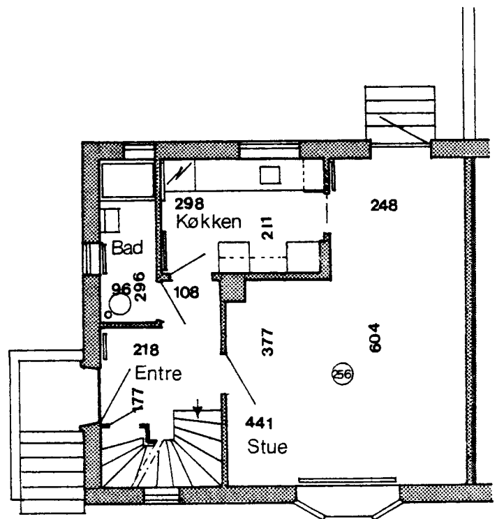
Stueplan
