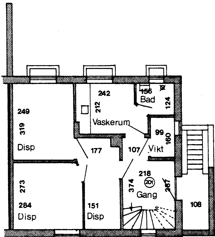
Kælderplan
