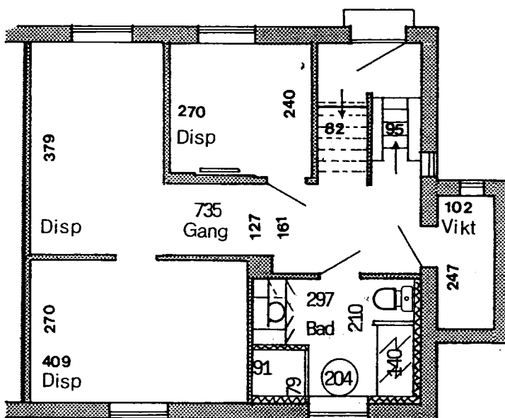
Kælderplan
