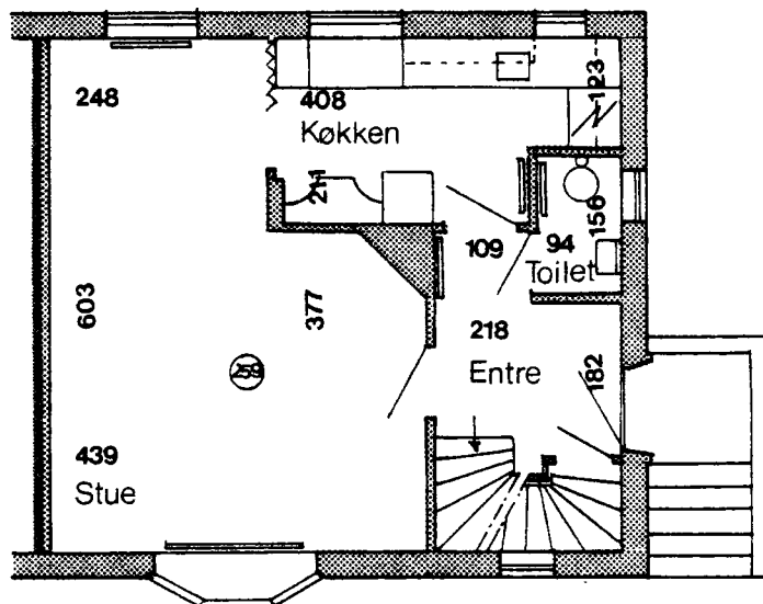
Stueplan
