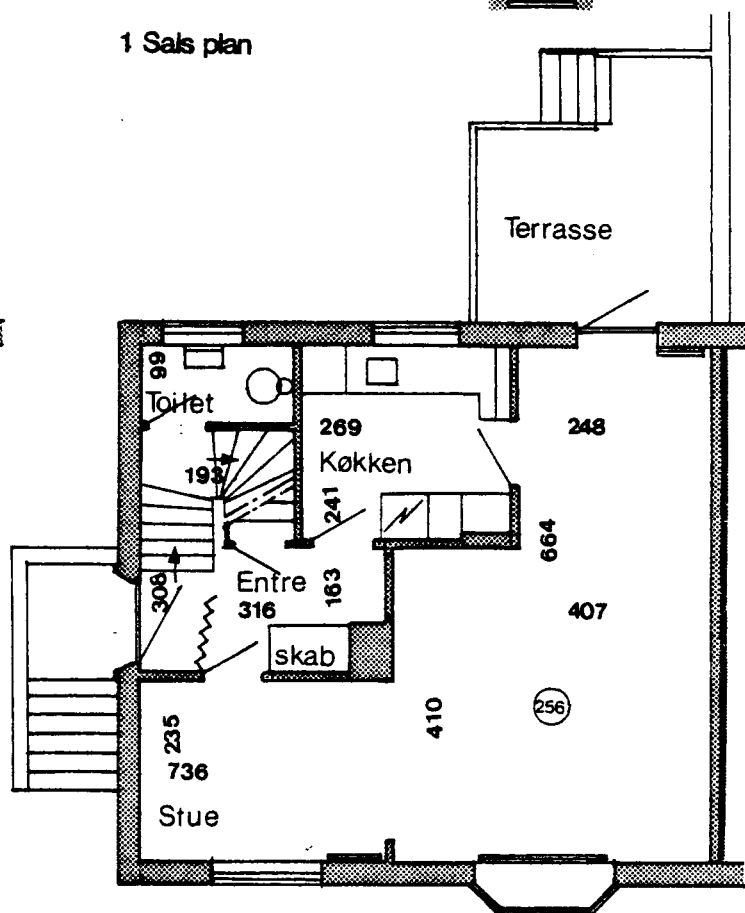
Stueplan
