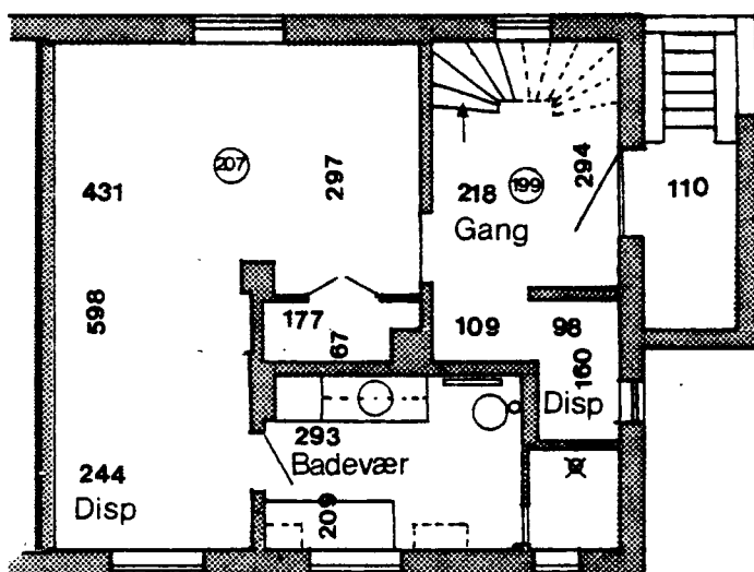
Kælderplan
