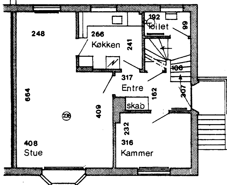
Stueplan
