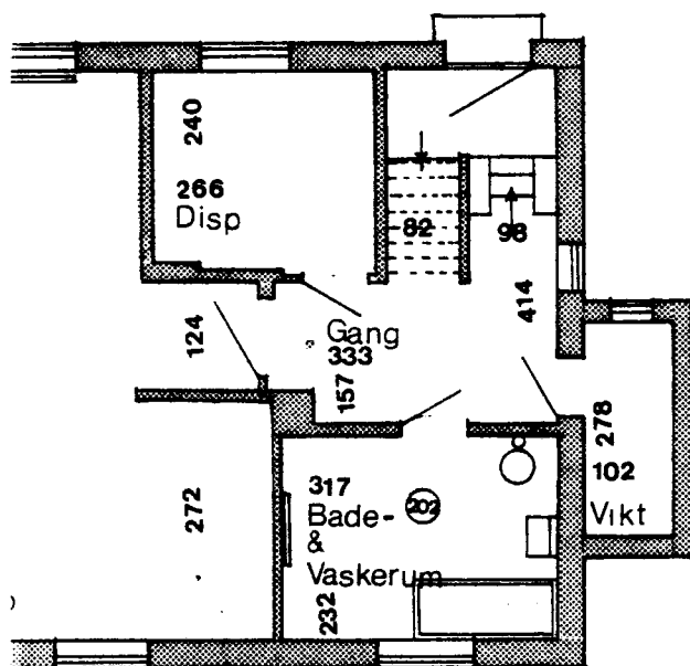
2. sal
