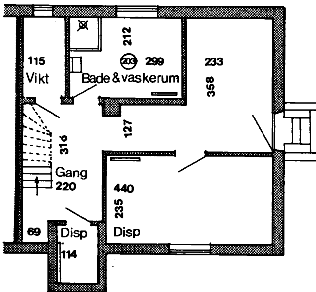
Kælderplan
