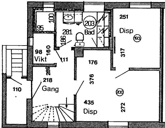
Kælderplan
