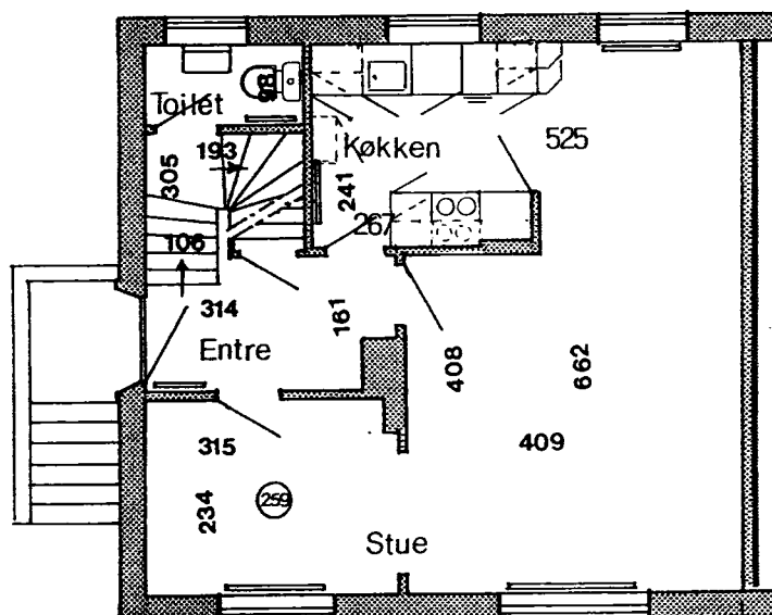
Stueplan
