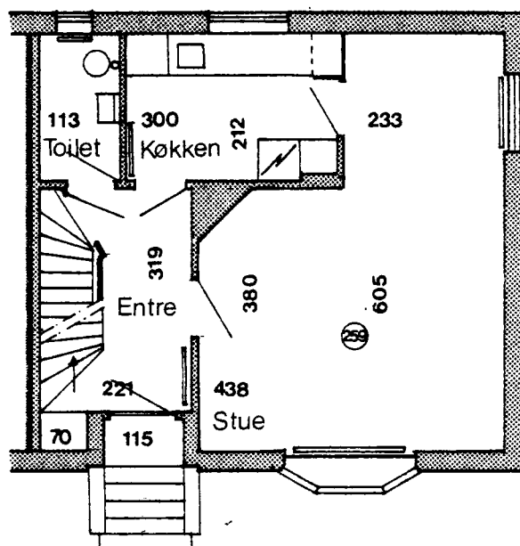
Stueplan
