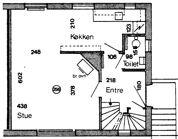
Stueplan
