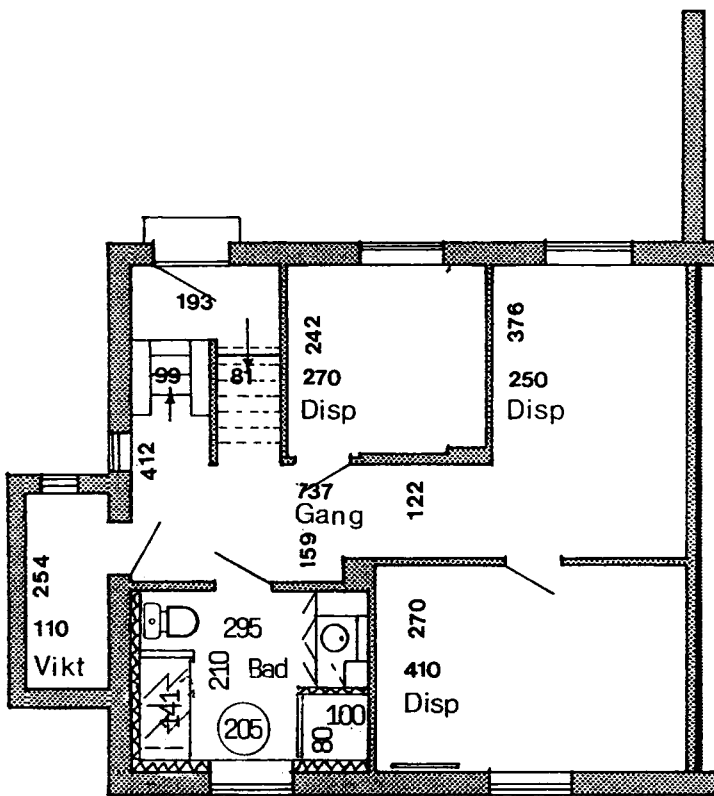
Kælderplan
