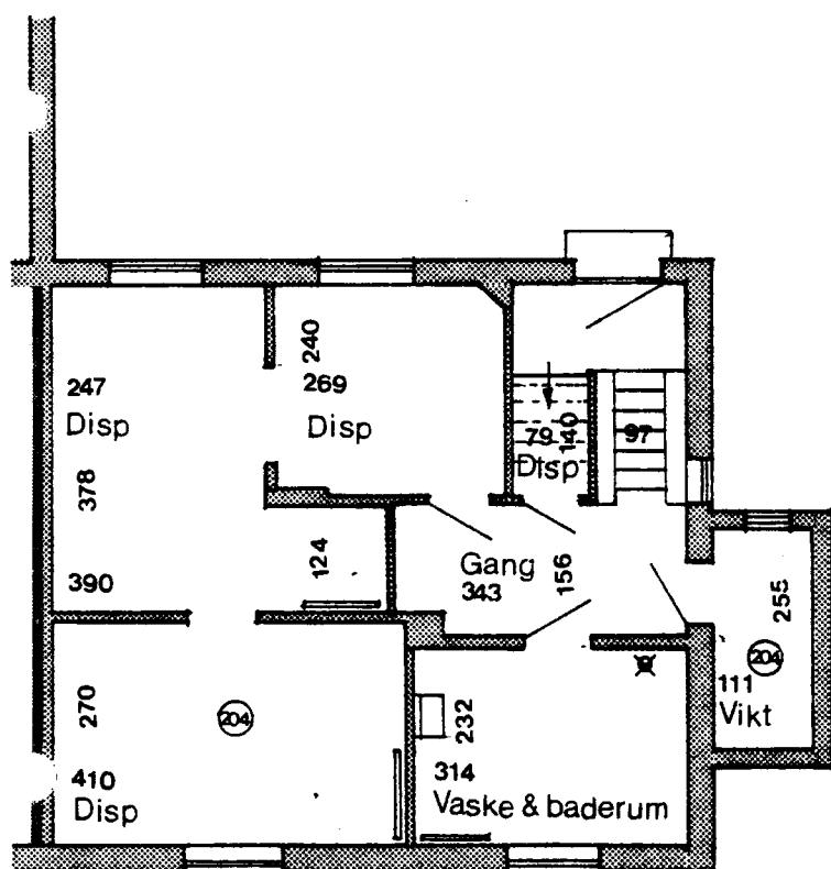
Kælderplan
