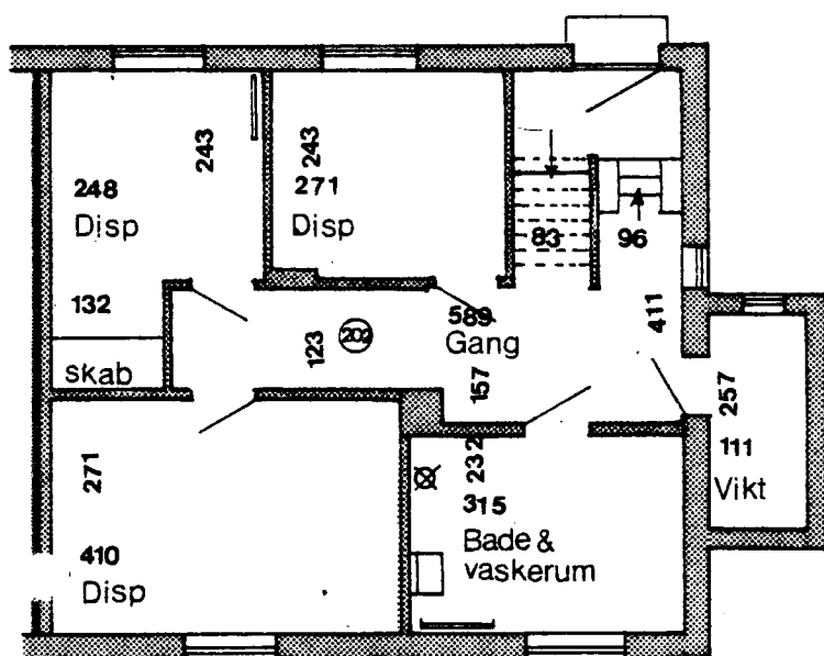
Kælderplan
