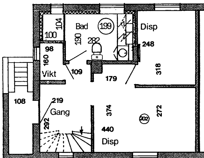
Kælderplan
