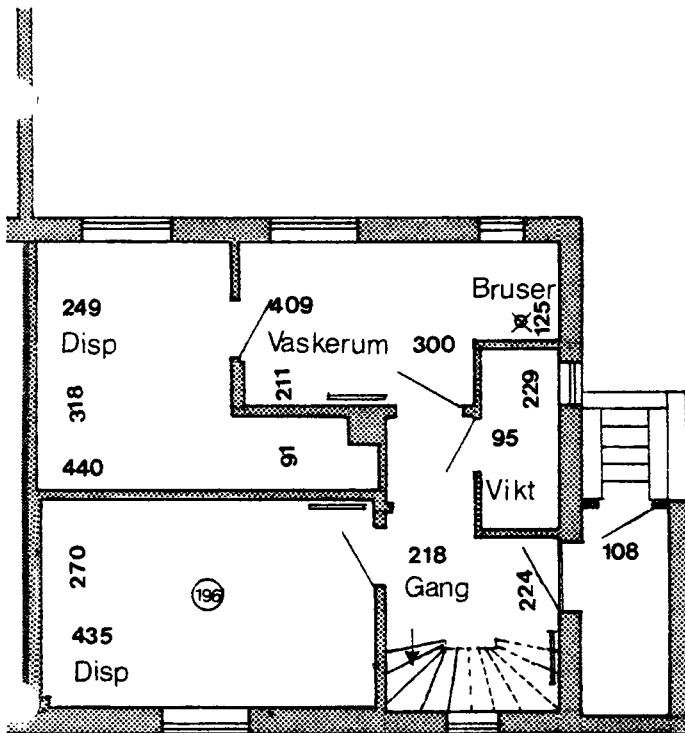
Kælderplan
