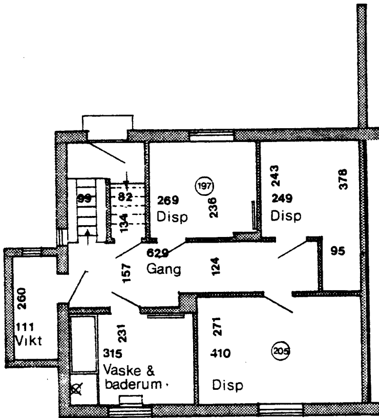
Kælderplan
