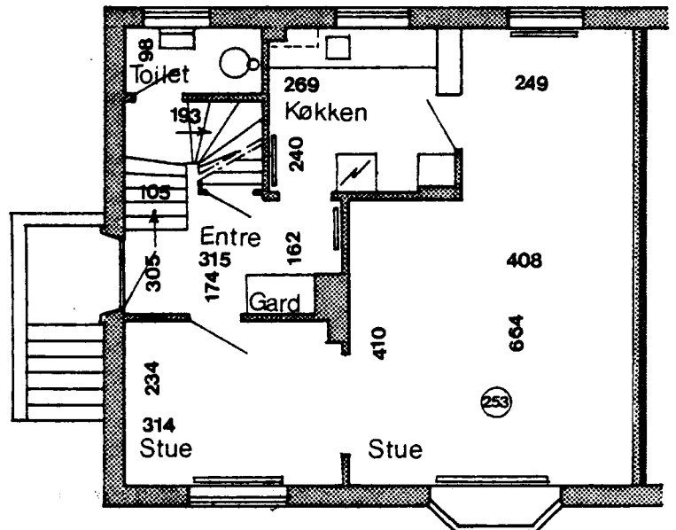
Stueplan
