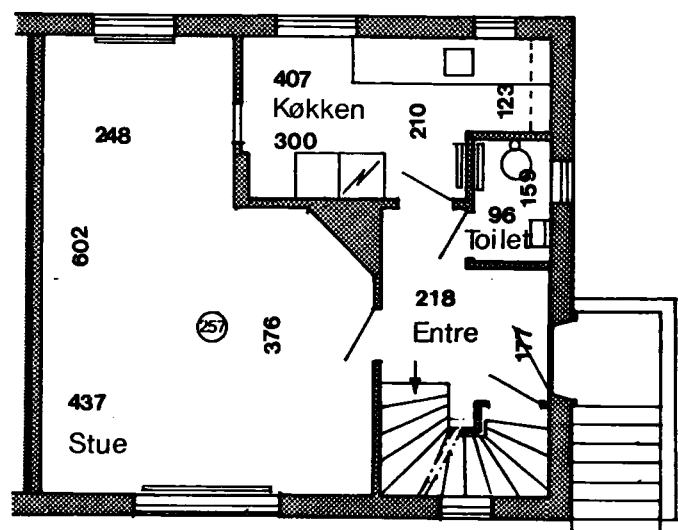
Stueplan
