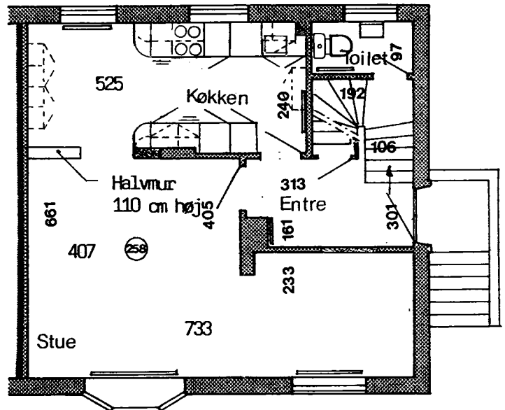
Stueplan
