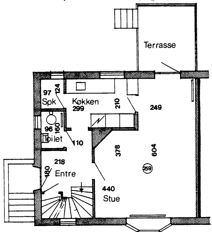
Stueplan
