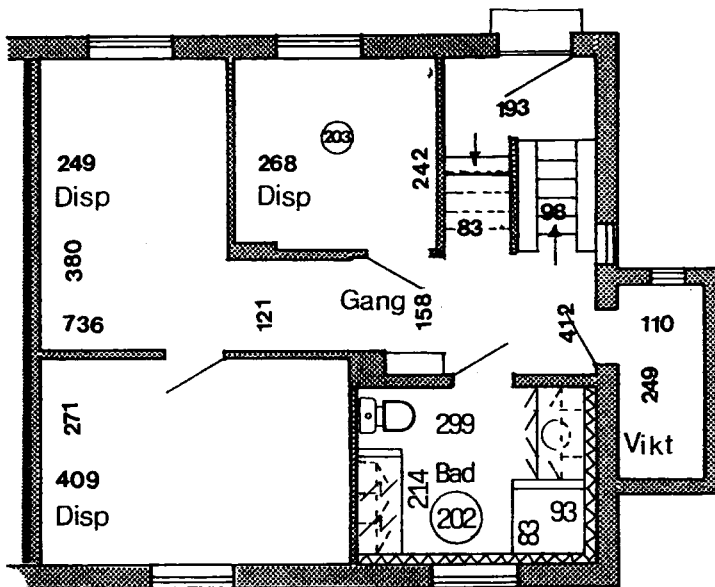
Kælderplan
