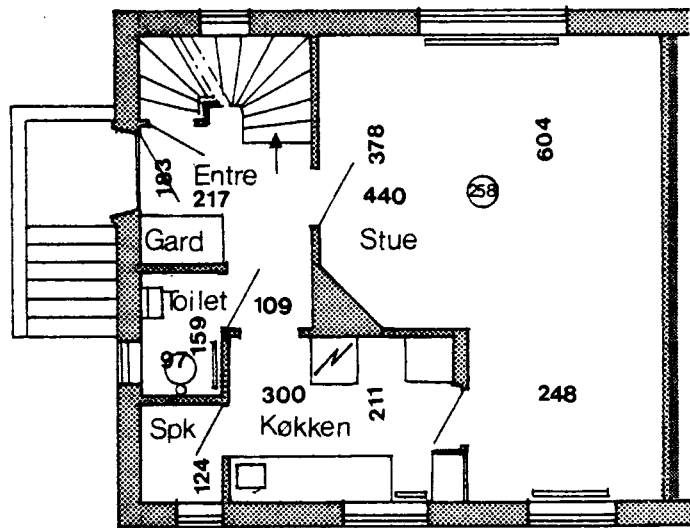
Stueplan
