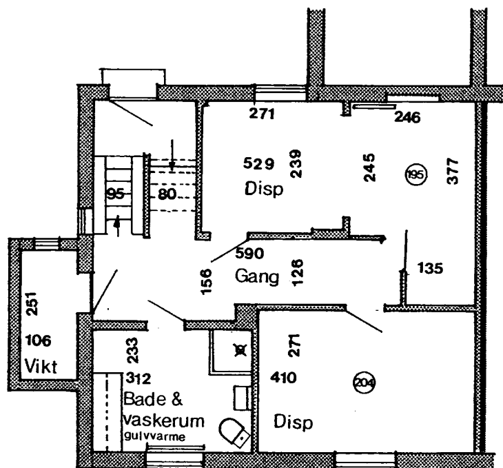
Kælderplan
