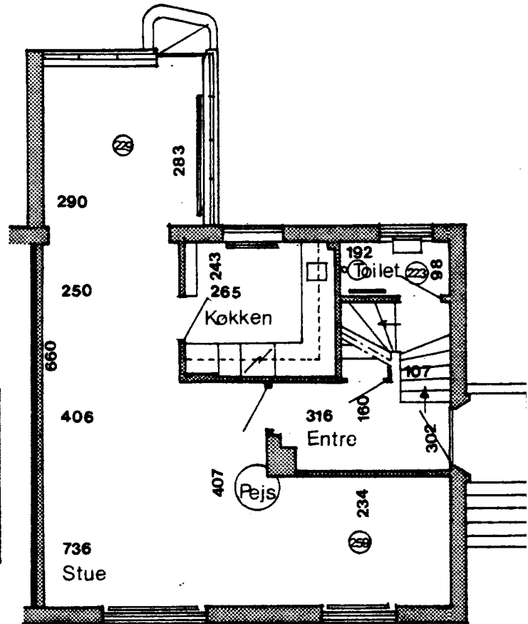
Stueplan
