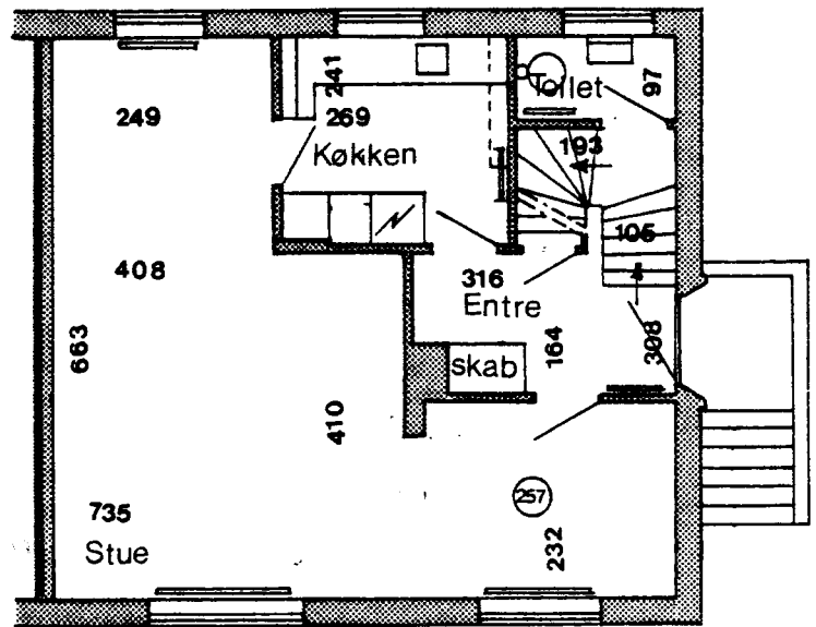
Stueplan
