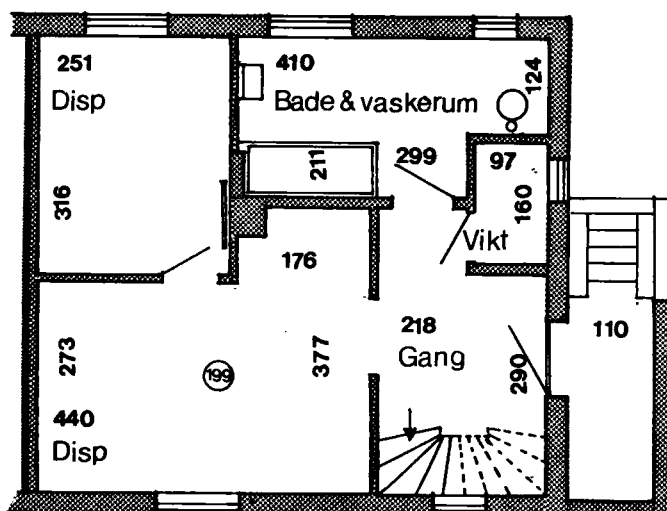
Kælderplan
