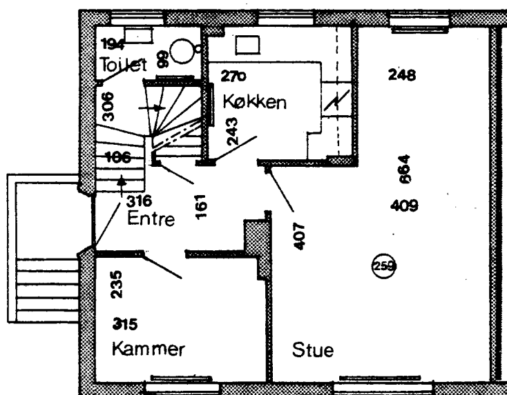
Stueplan
