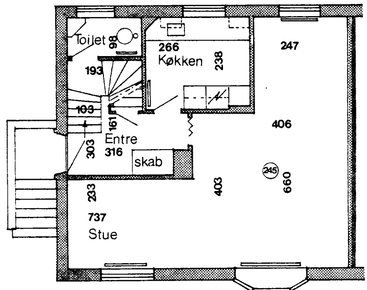
Stueplan
