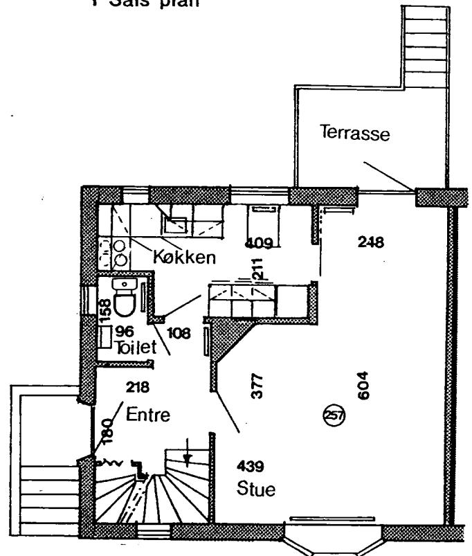
Stueplan
