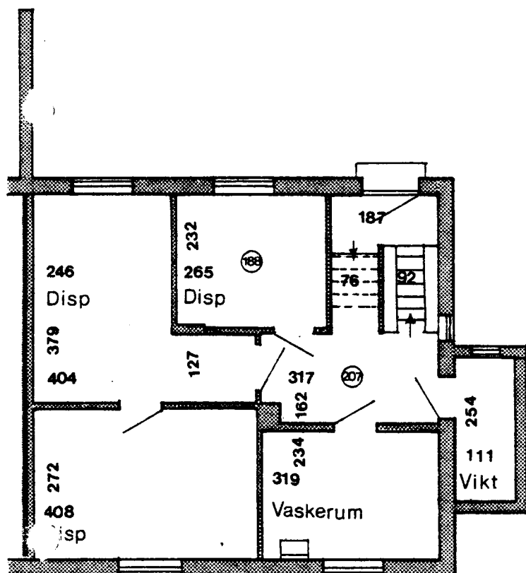
Kælderplan
