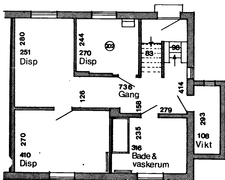
Kælderplan
