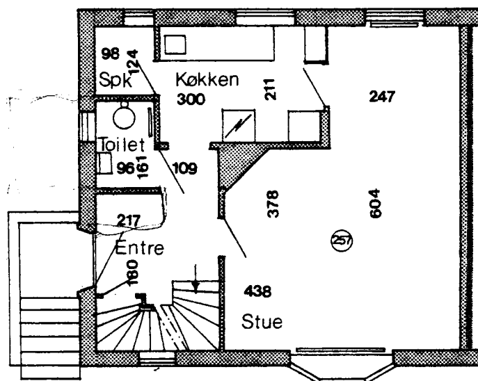
Stueplan
