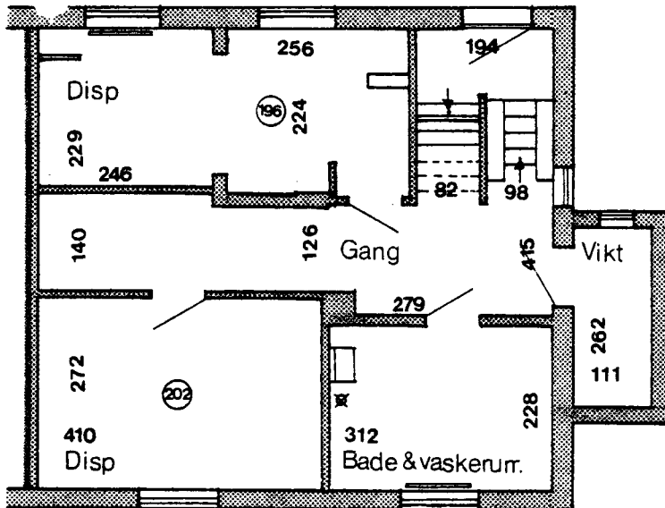
Kælderplan
