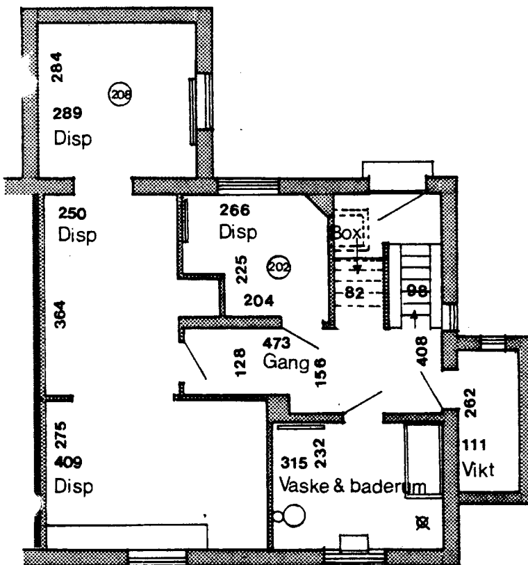
Kælderplan
