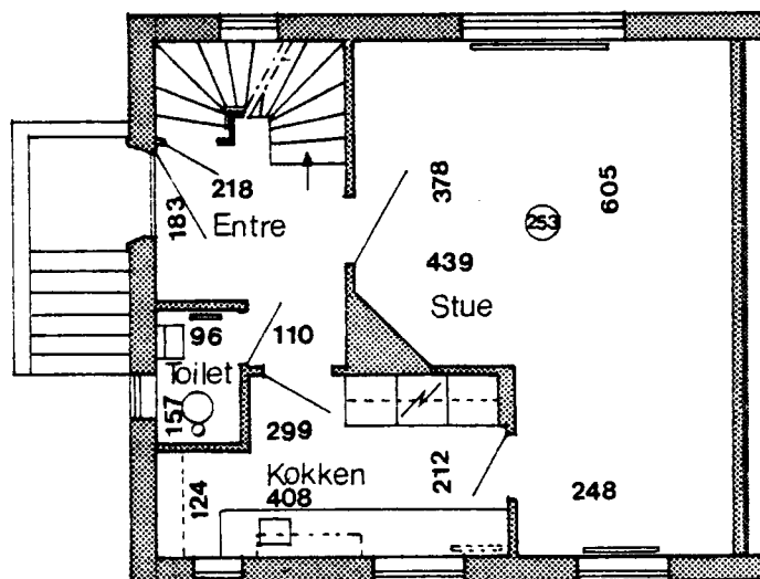
Stueplan
