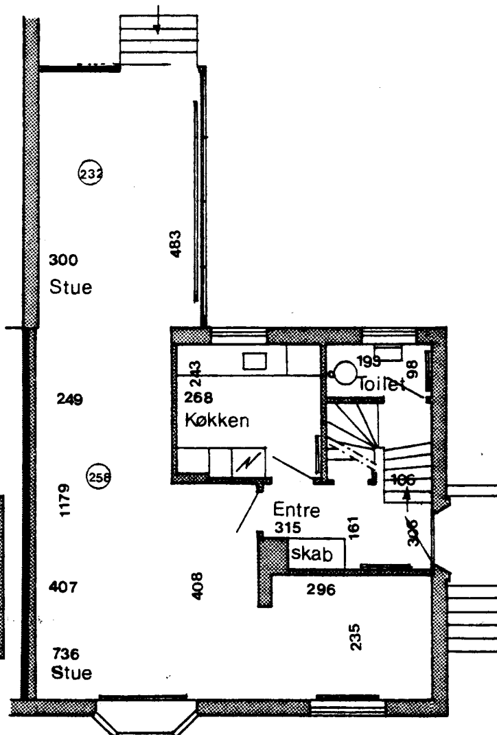
Stueplan
