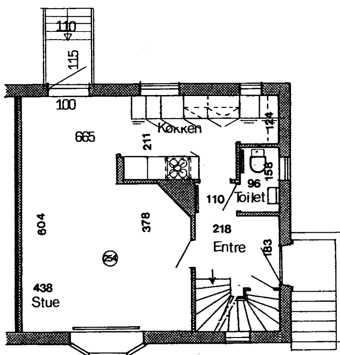
Stueplan
