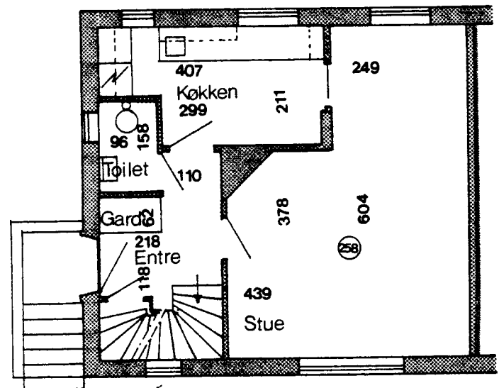
Stueplan
