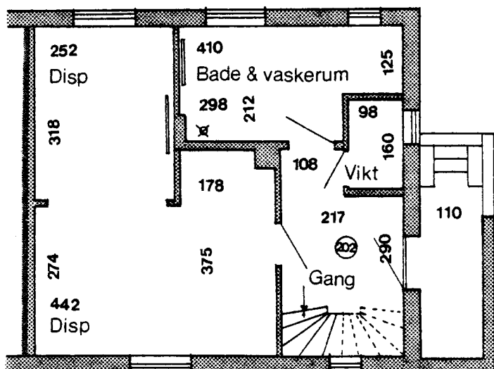
Kælderplan
