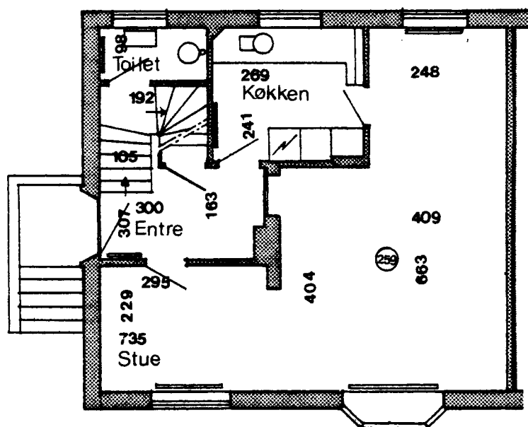
Stueplan
