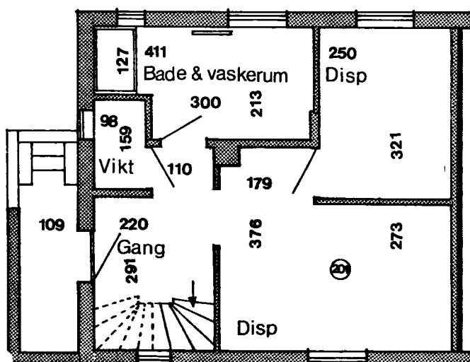
Kælderplan
