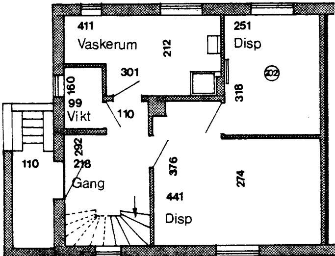
Kælderplan
