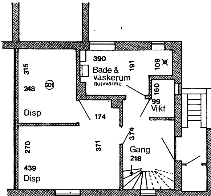
Kælderplan
