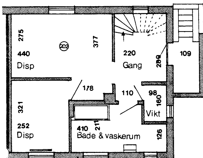
Kælderplan
