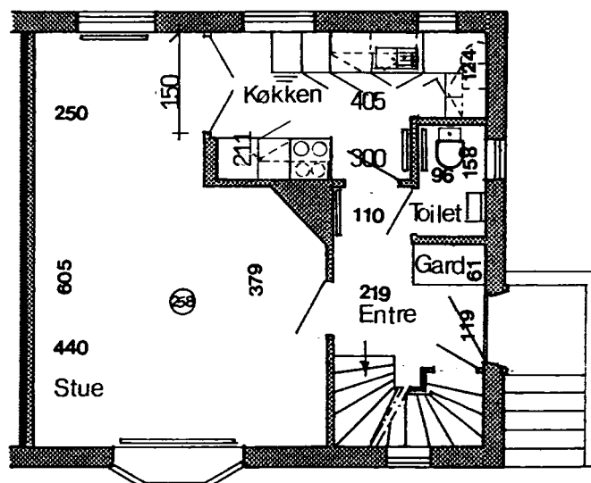
Stueplan
