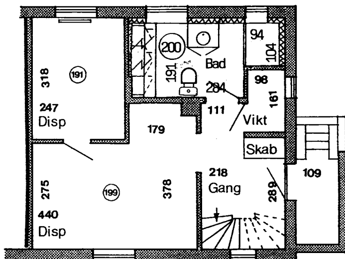
Kælderplan
