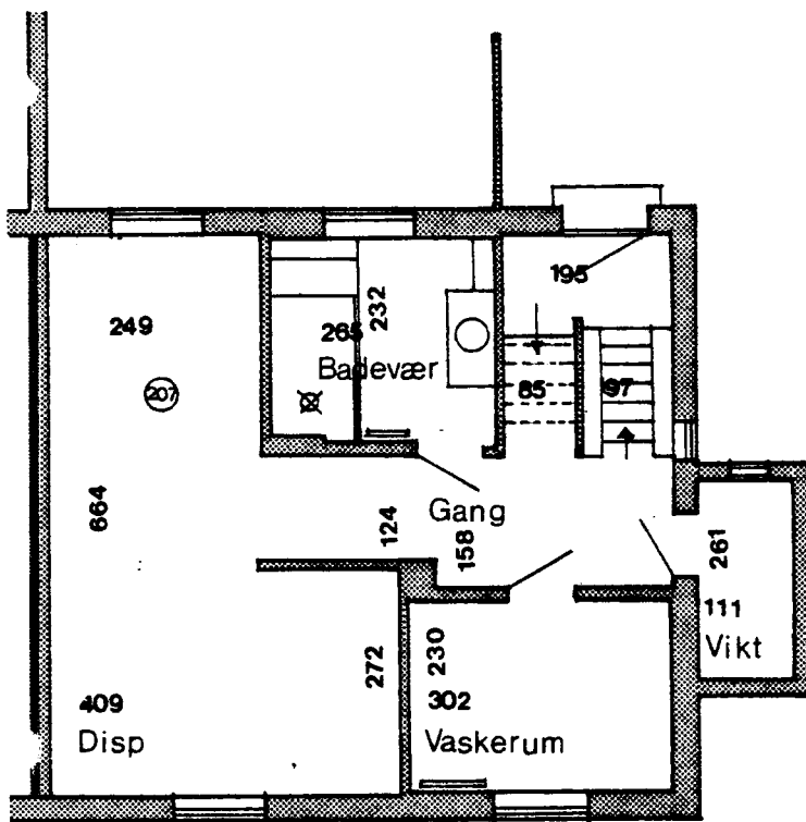
Kælderplan
