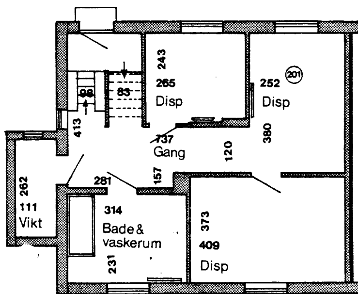
Kælderplan
