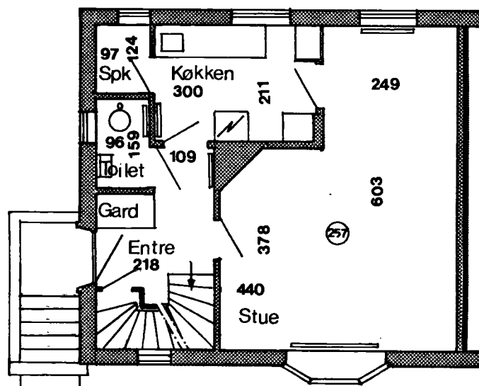
Stueplan
