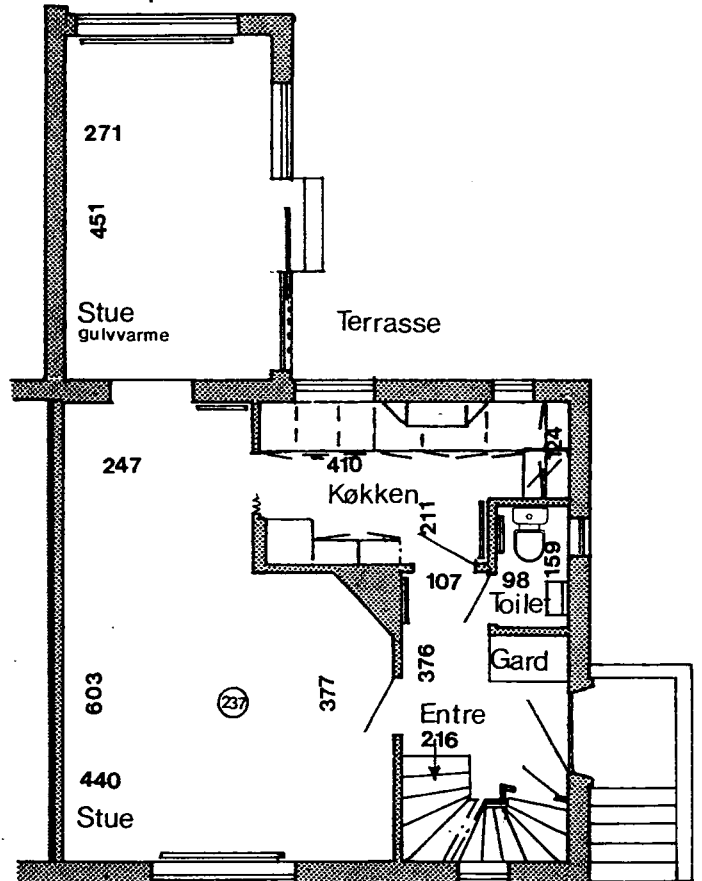
Stueplan
