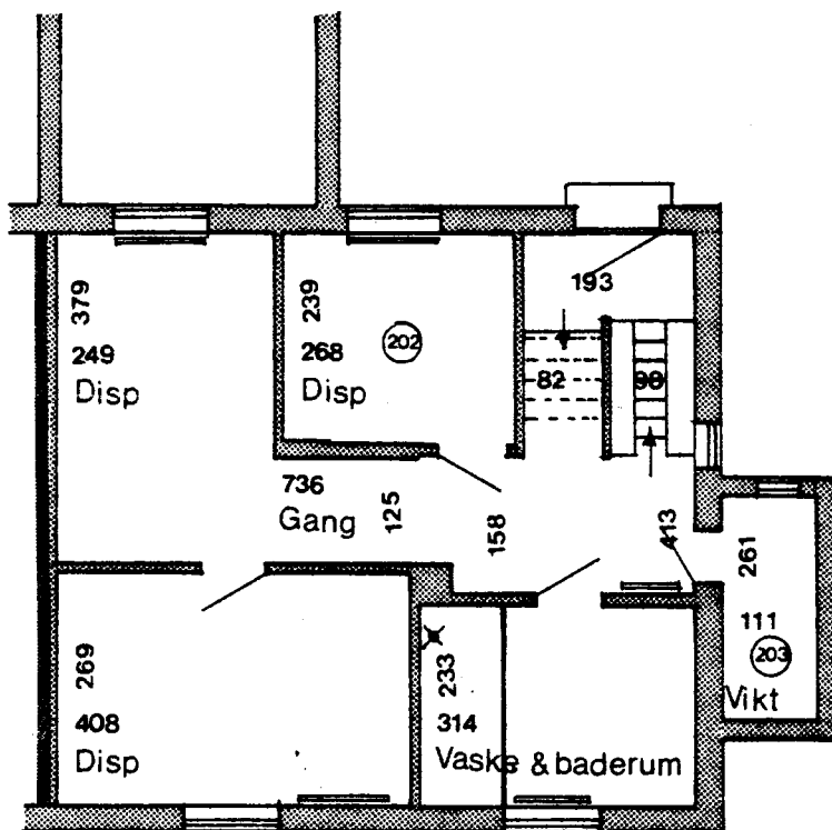
Kælderplan
