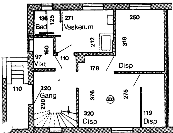
Kælderplan
