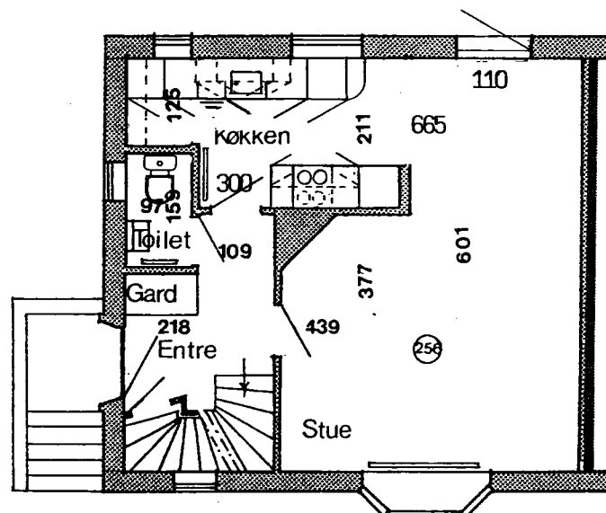
Stueplan
