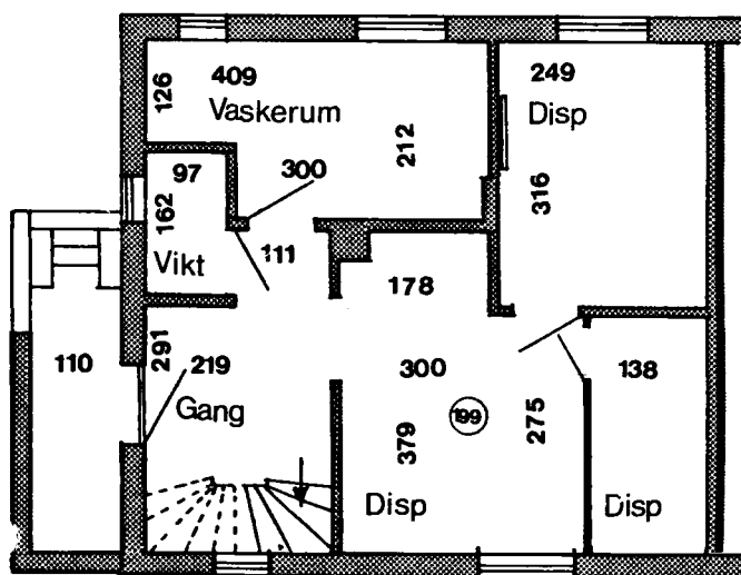
Kælderplan
