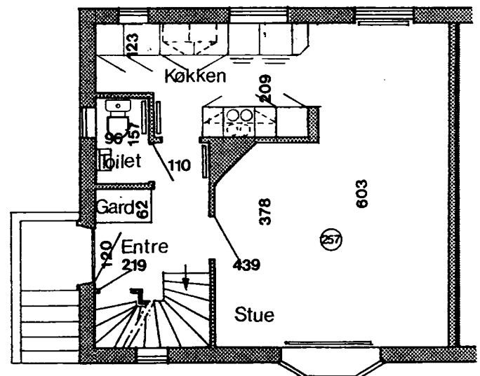
Stueplan
