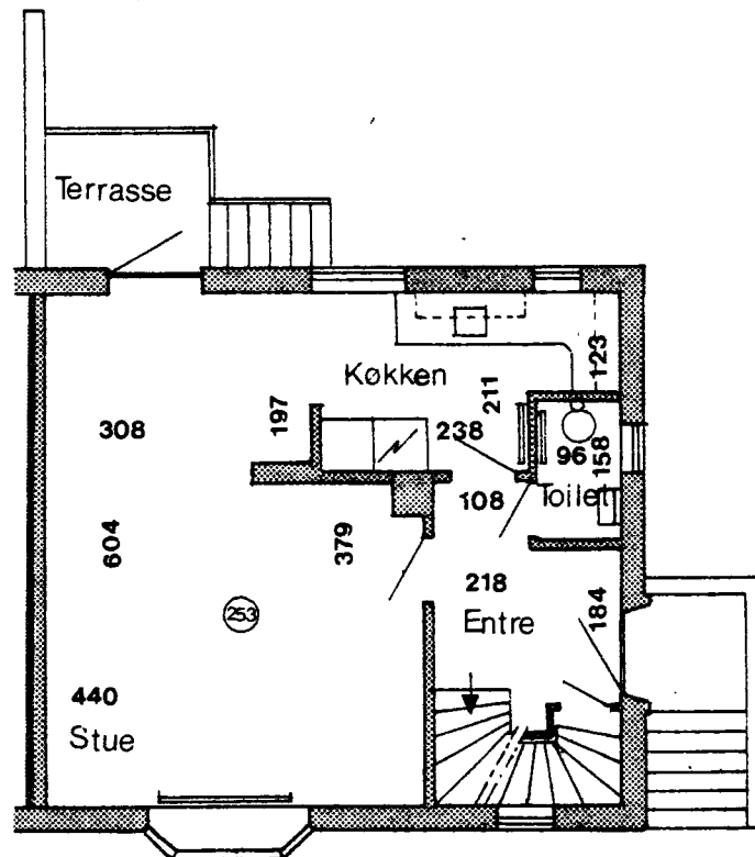
Stueplan
