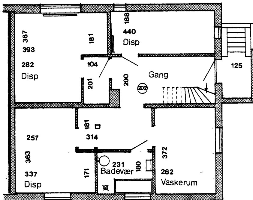
Kælderplan
