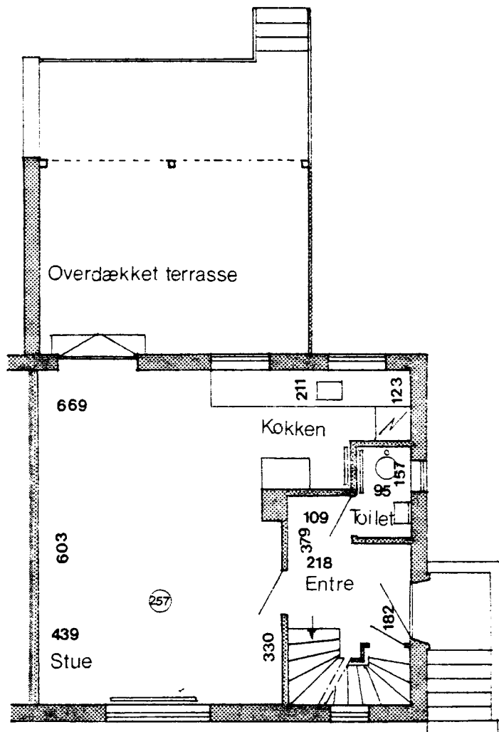
Stueplan
