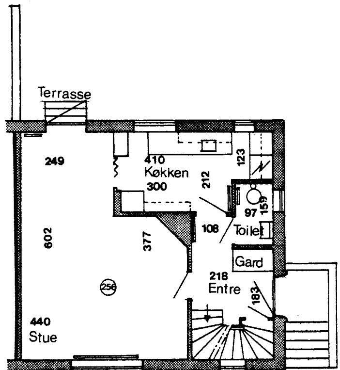
Stueplan
