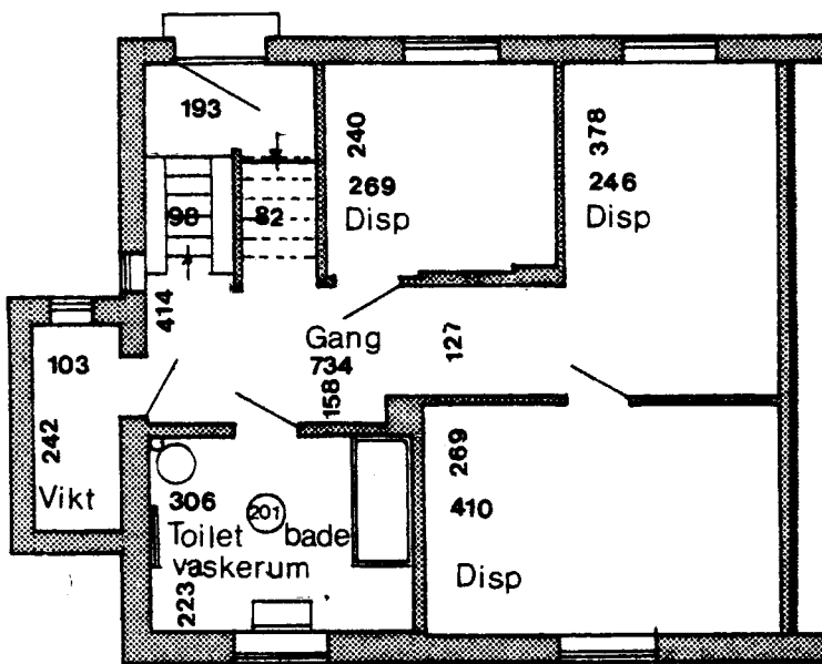
Kælderplan
