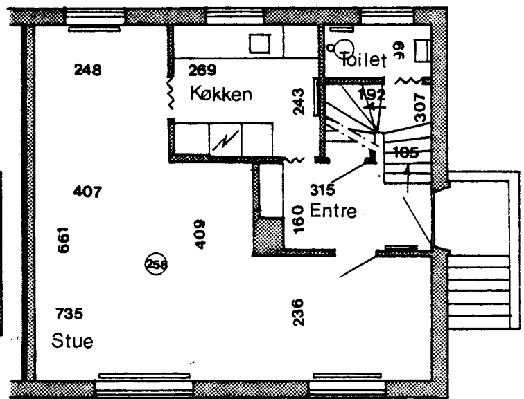
Stueplan
