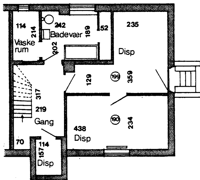
Kælderplan
