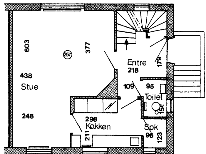
Stueplan
