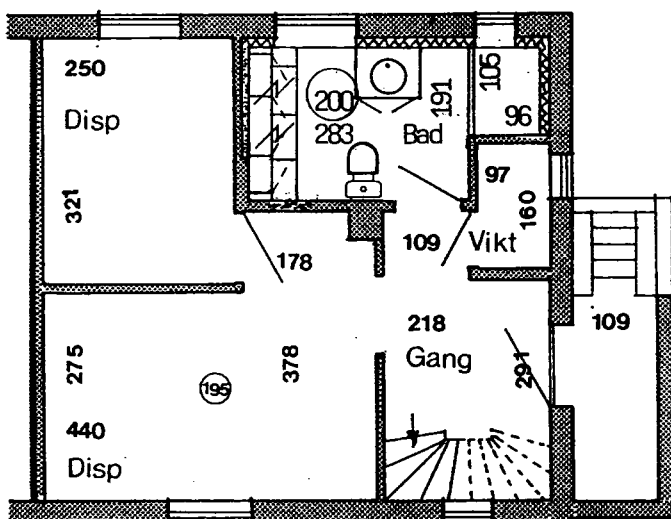
Kælderplan
