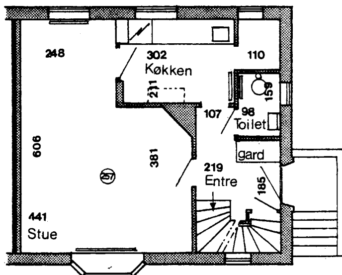
Stueplan
