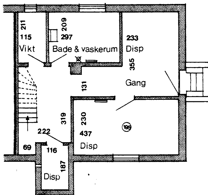
Kælderplan
