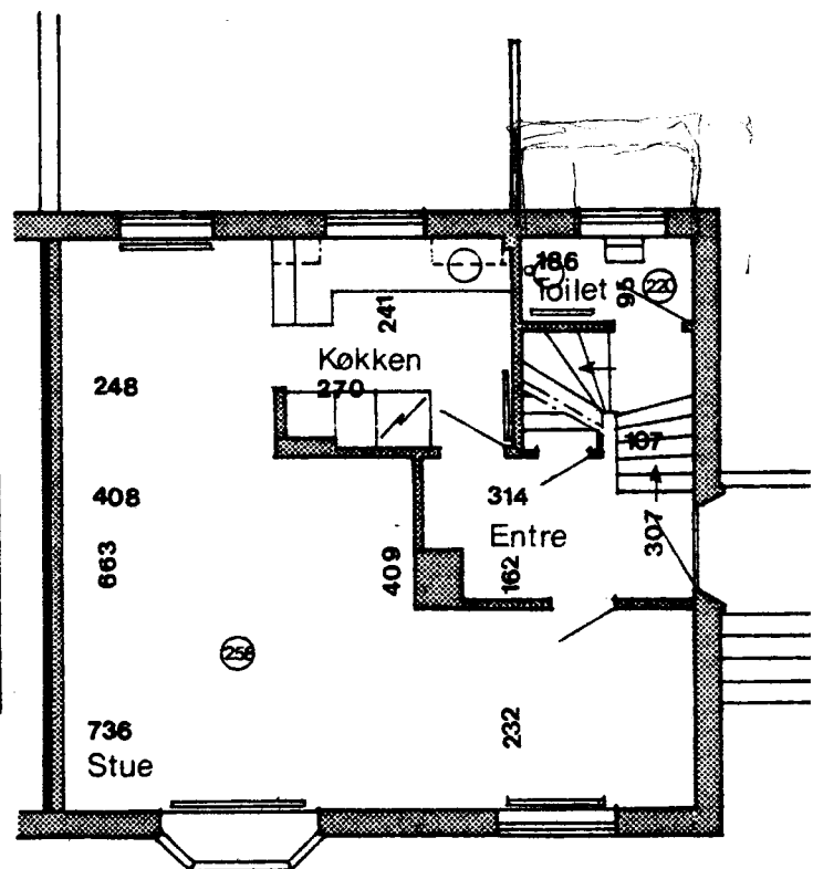
Stueplan
