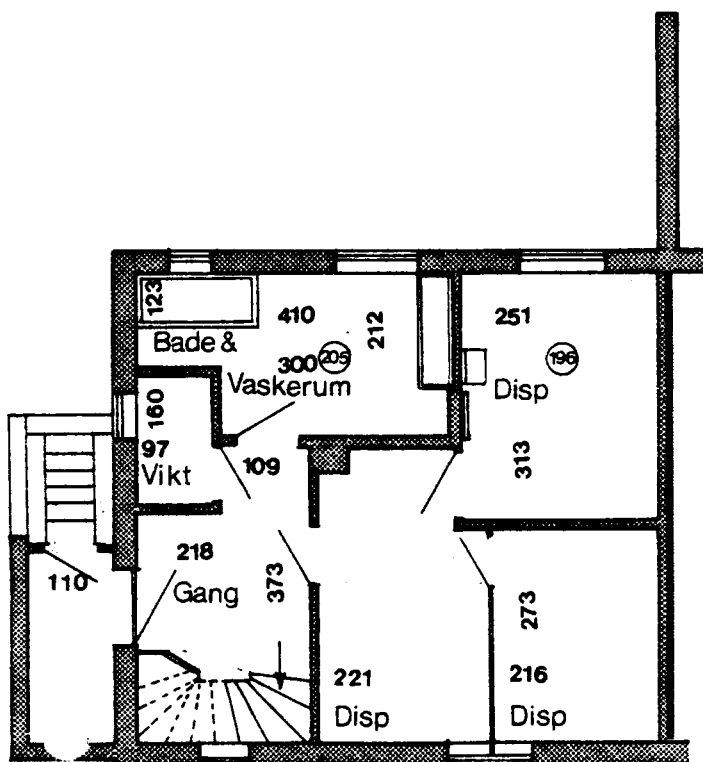
Kælderplan
